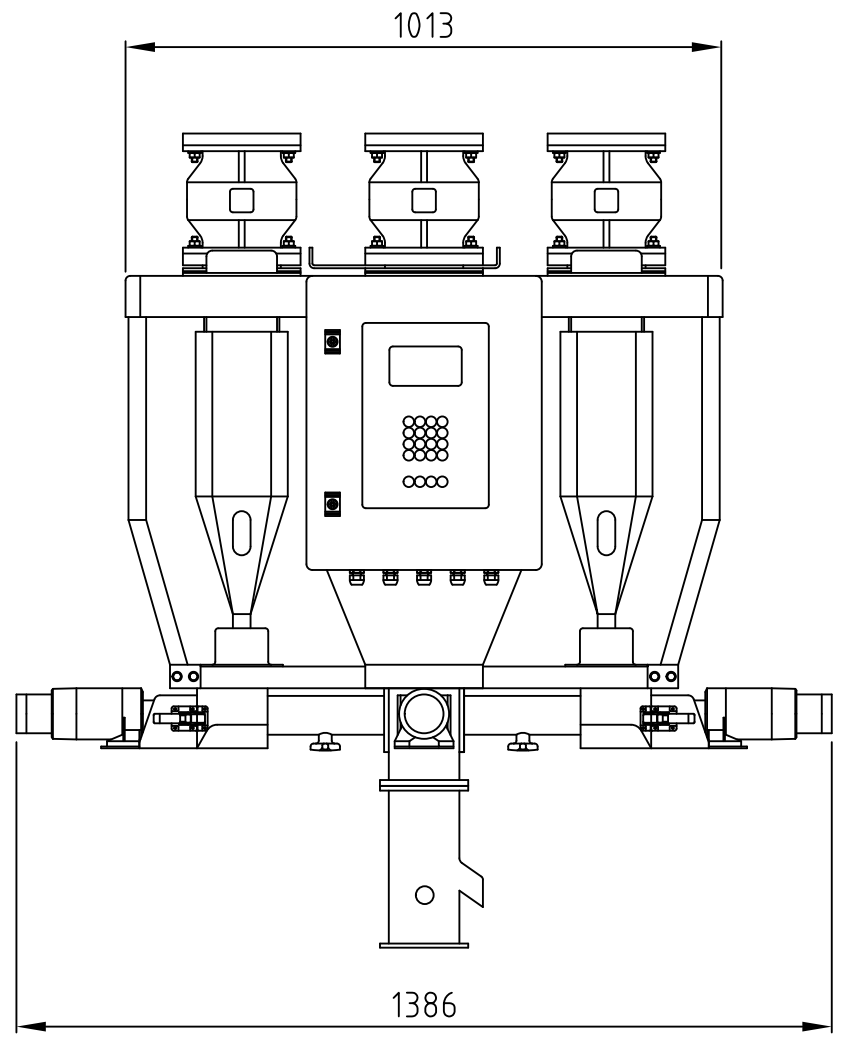
END ELEVATION
